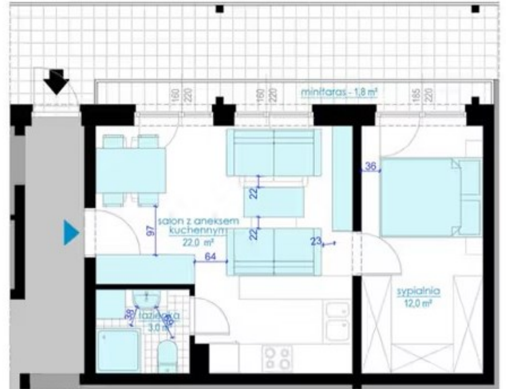
Rzut z normalnej wielkości meblami
