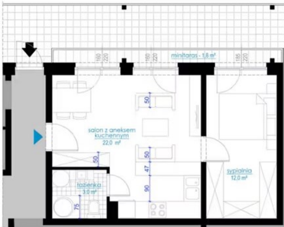
Rzut mieszkania od dewelopera
